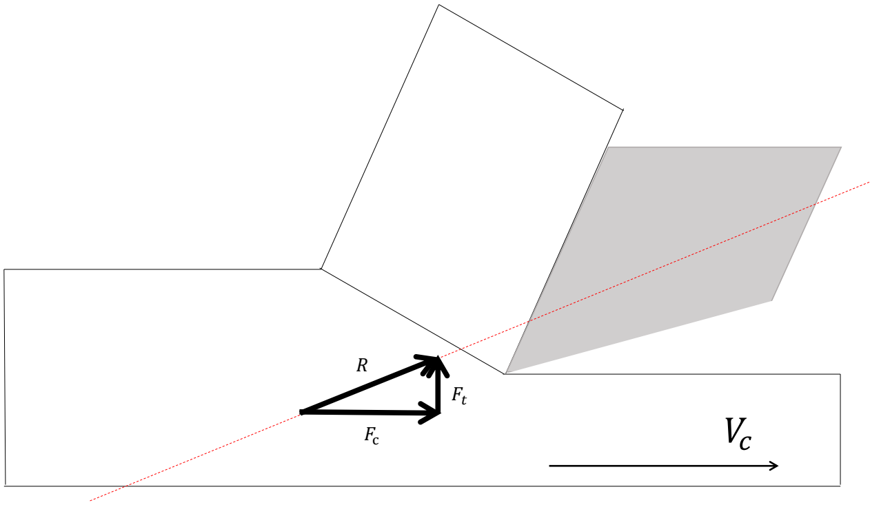
図：切削における合力 R の分解（見方①）.
