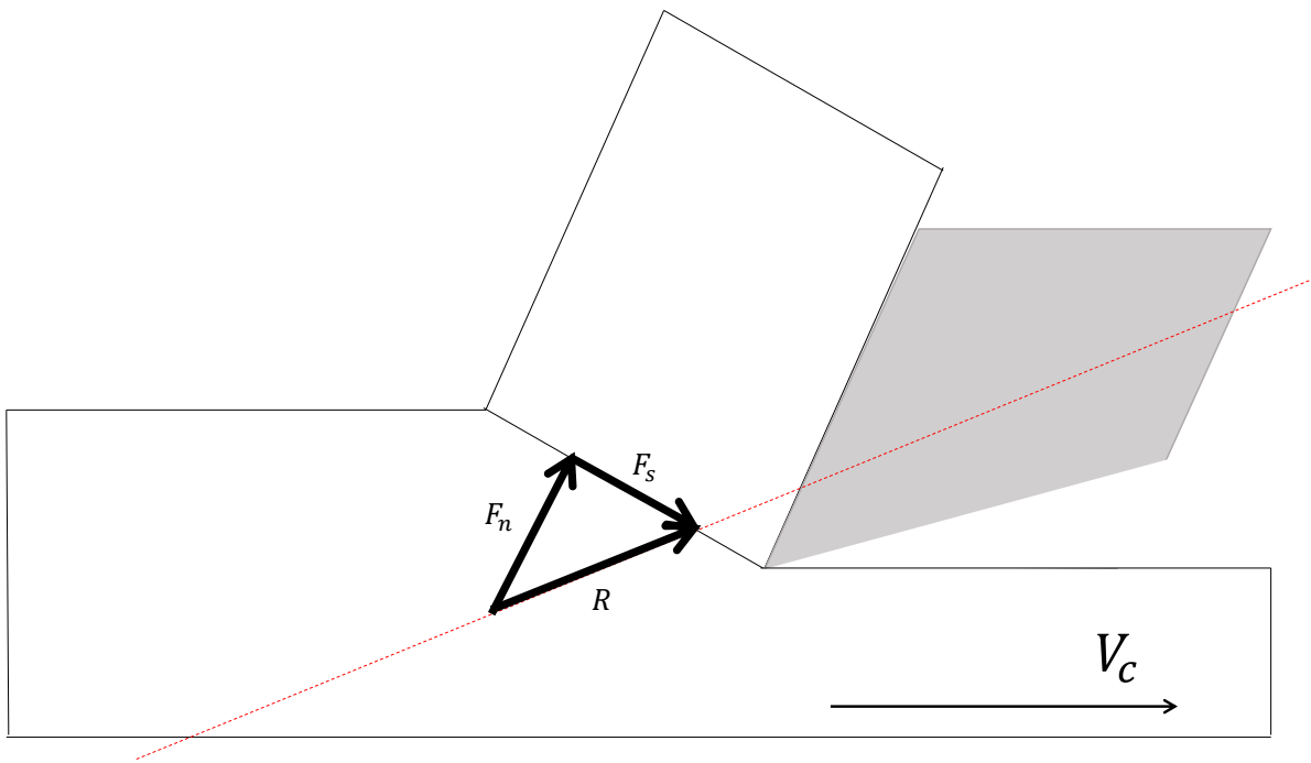
図：切削における合力 R のせん断面における影響（見方②）.
